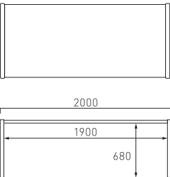
BEBR-TD200R W2000 D884 H725
