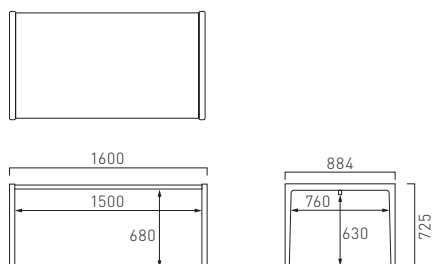
BEBR-TD160R W1600 D884 H725
